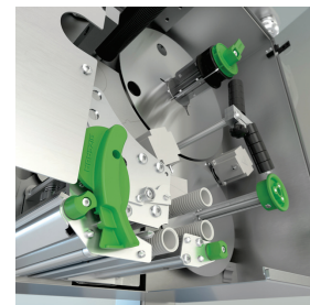
GLM Etikettierer für Plug-In®-Label
