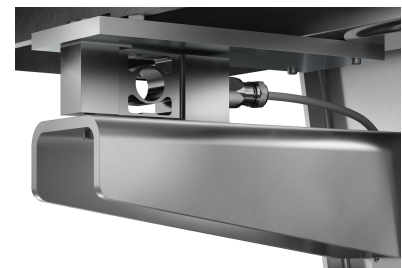
Detail Wägezelle
